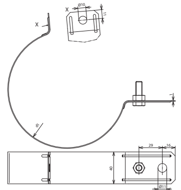
Maßbild RRS 120 B11 CU
