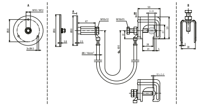
Maßbild UES 16 L600 VK RD8 28 FL30 EFP
