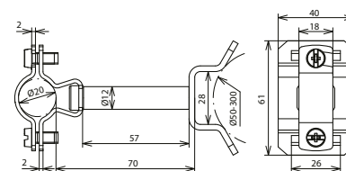
Maßbild LH ZS 20 EX P70 SBB V2A
