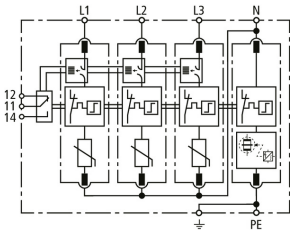
Prinzipschaltbild DG M TT ACI 385 FM
