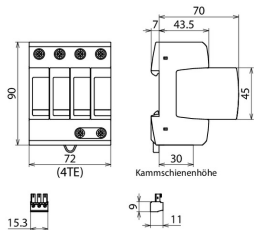
Maßbild DG M TT ACI 385 FM
