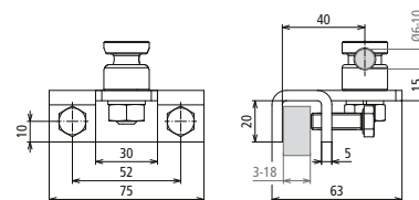
Maßbild AK 6.10 KSV FER W KBF3 18 V2A
