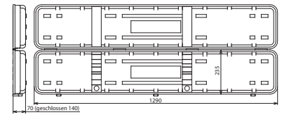
Maßbild KKL PHE L
