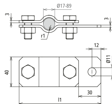
Maßbild ERS 42 AB11 STTZN
