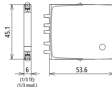
Maßbild BCO MOD ML2 BE 180
