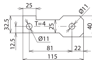
Maßbild AB EXFS IF3 G 11
