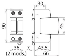
Maßbild DG MU CGD 480 3W+G
