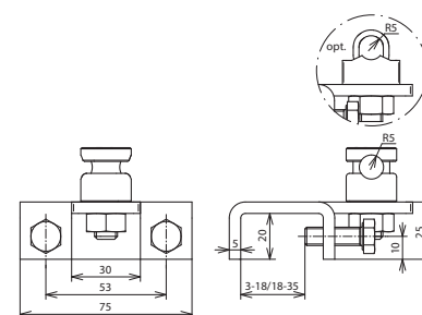
Maßbild AK 6.10 KSV W KBF18 35 V2A
