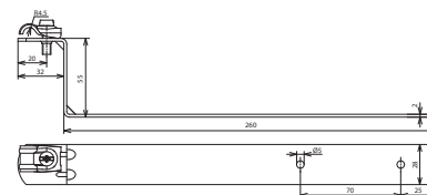
Maßbild DLH DQ 6.10 H55 L260 STTZN
