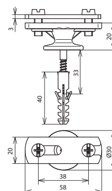
Maßbild FBH ZS 30 IGM8 KD8X40STTZN ZG
