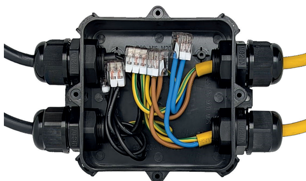
Beispielverdrahtung
