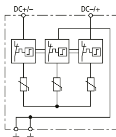
Prinzipschaltbild DCB YPV 1500
