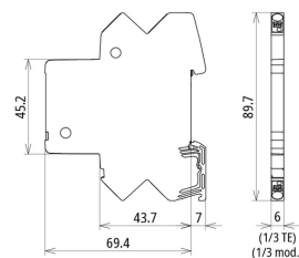
Maßbild BCO CL2 BD HF 5
