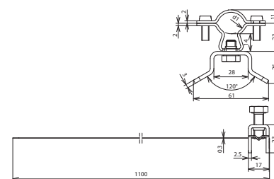
Maßbild LH ZS 20 23 SB50.300 V2A
