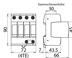
Maßbild DG M TT 385
