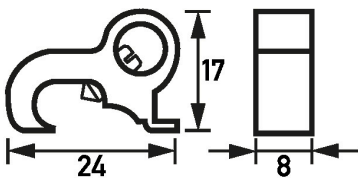
Maßzeichnung Gruppenansicht
