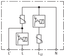
Prinzipschaltbild DCOR L 2P SN1864
