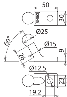
Maßbild KFP 25 S AL 12
