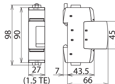
Maßbild DG SE DC 242
