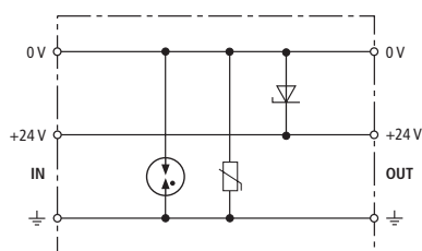
Prinzipschaltbild BVT AVD 24
