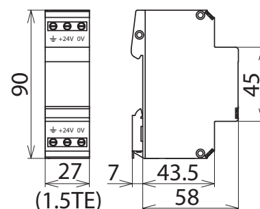
Maßbild BVT AVD 24
