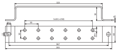
Maßbild ES 2X6 ASB11 V2A
