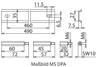
Maßbild MS DPA
