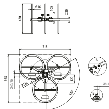
Maßbild DBS KB D40.50 RA220 STTZN
