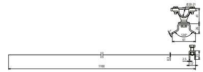
Maßbild LH ZS 20 SB50.300 PA V2A
