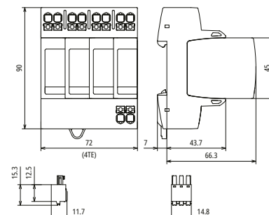
Maßbild DG MP TNS 150 FM
