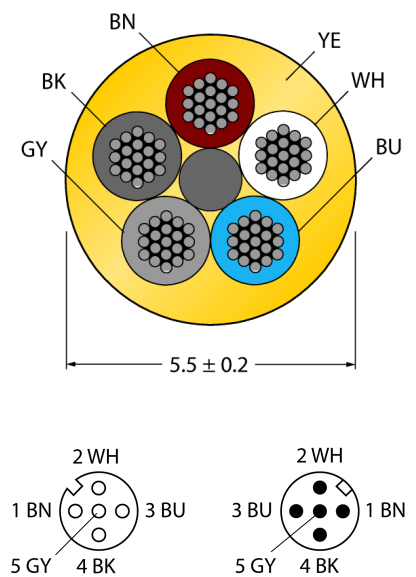
Leitungsquerschnitt
