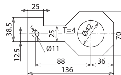
Maßbild AB EXFS IF3 G 42
