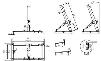
Maßbild MDH D48 VB550.900 V2A
