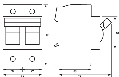
Maßzeichnung Sicherungslasttrennschalter Coron 2 Do-63-2
