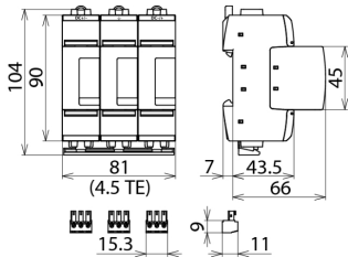
Maßbild DG ME YPV SCI1500 FM
