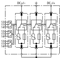
Prinzipialschaltbild DG ME YPV SCI1500 FM
