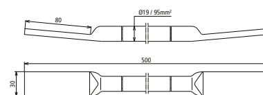
Maßbild D BEB 10 / EBS 15-03-19
