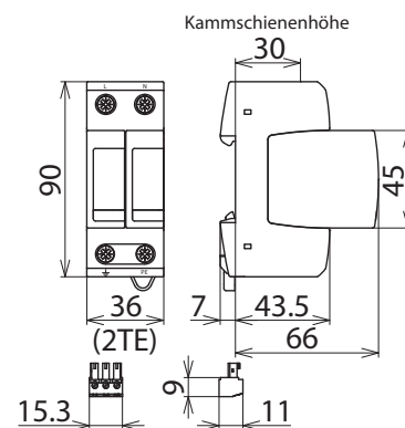
Maßbild DG M TT 2P 275 FM
