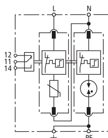
Prinzipialschaltbild DG M TT 2P 275 FM
