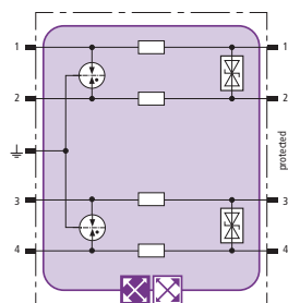
Prinzipschaltbild BXT ML4 BD HF 24
