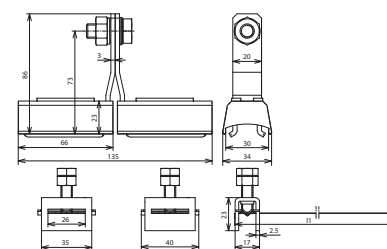
Maßbild EX BRS 90
