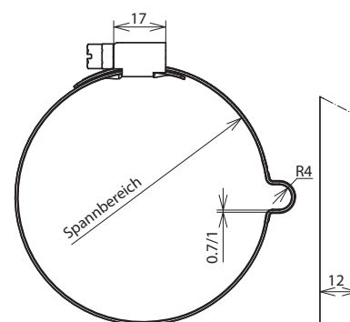
Maßbild LH 8 SB80.100 SCG GALCU
