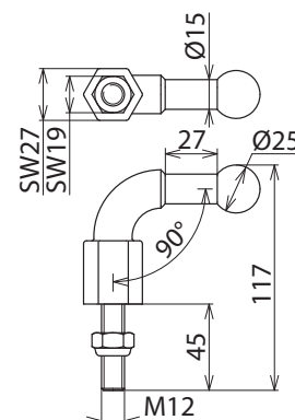
Maßbild KFP 25 W90 M12 45SSM
