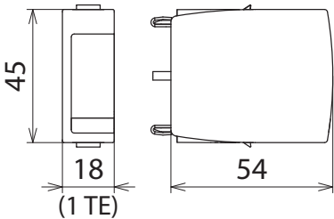
Maßbild DG MOD ACI 275
