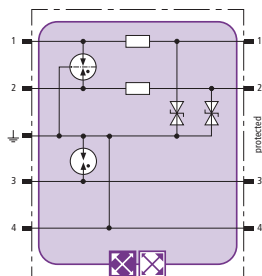
Prinzipschaltbild BXT ML2 BE S 5
