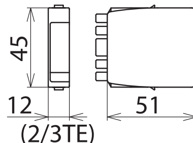
Maßbild BXT ML2 BE S 5
