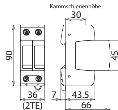
Maßbild DG M TT 2P 275
