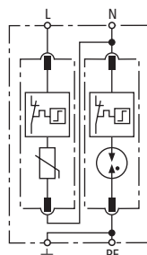
Prinzipialschaltbild DG M TT 2P 275
