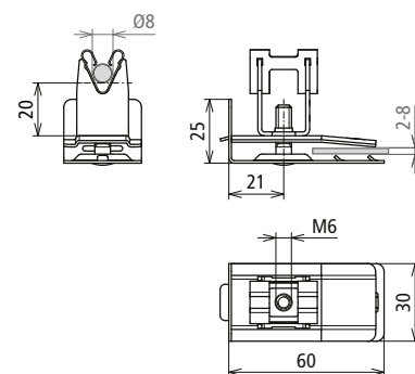
Maßbild DLH DG 8 H20 KB2.8 KU V2A
