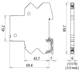
Maßbild BCO CL2 BE 24
