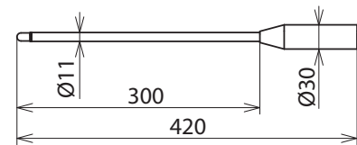
Maßbild PSO M8 PHE
