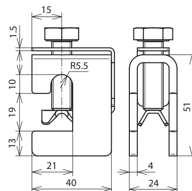
Maßbild AK 6.10 DS KBF5 18 V2A
