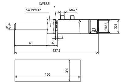
Maßbild AE BO10 KF HVI 60 V2A
