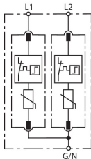
Prinzipialschaltbild DG MU CGD 240 3W+G
