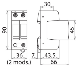
Maßbild DG MU CGD 240 3W+G
