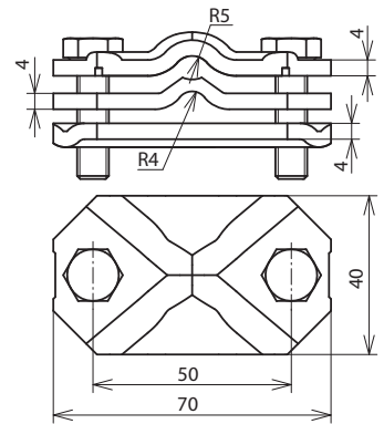
Maßbild VTK 5.10 FL30.40 ZP STTZN
