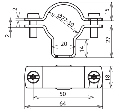
Maßbild LH ZS 27 B5.5X10 V2A
